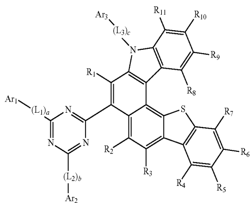
Formula 2e
