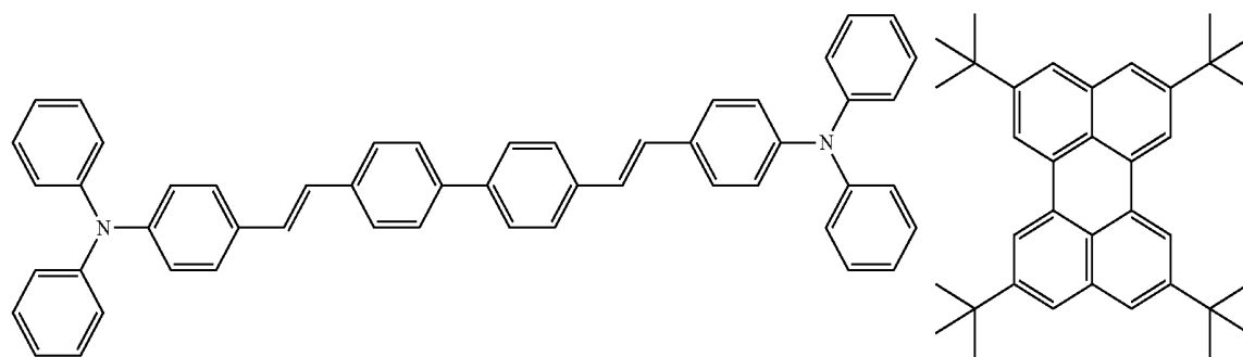
DPAVB
