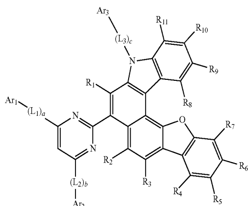
Formula 2e
